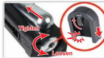
マガジン底版を叩いて六角レンチを使用してください。六角レンチで下部のカートリッジトレイを外して、CO2カートリッジを取り付けます。マガジンを取り付け、トレイを閉めます。
