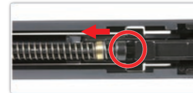
リコイルスプリングガイドを前方に押し当ててください。
