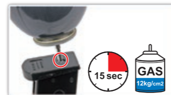
注入バルブに、ガスボンベのノズルを合わせる。
